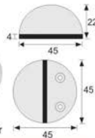
TCH-8404 Glass Door Stopper
