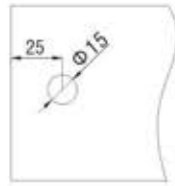
Size & Cutout Details for TCH-8438, TCH-8438 A & TCH-8438 R U Connector
