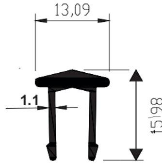
20142 WT KG/12FT=0.600
