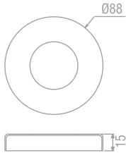
MWCC - 42.4/50 (S.S. 316) AMWCC - 42.4/50 (S.S. 304) Wall Cover Cap
