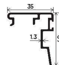
Universal Clip Section Number : V-2521 Weight (kg/mt) : 0.393
