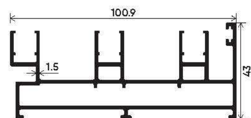
Premium Type Section Number : V-2504 Weight (kg/mt) : 1.676
