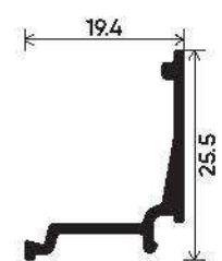
CLIP
