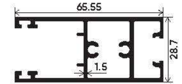
Top & Bottom S. G. Shutter Section Number : V-3112 Weight (kg/mt) : 1.079
