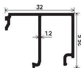
CLIP
