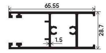
Top & Bottom DGU Shutter Section Number : V-3116 Weight (kg/mt) : 1.079
