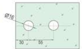
HGP -109 GR Door Hinge - Grey
