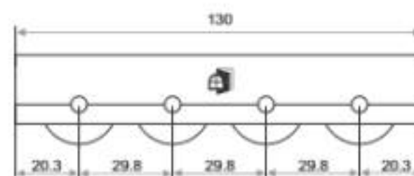
AI29130U
