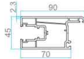
AP 305 A SLIDING DOOR SASH
