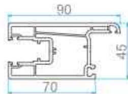
AP 305 SLIDING DOOR SASH
