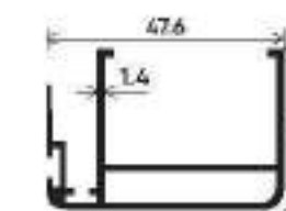
INTERLOCK
