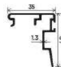
INTERLOCK CLIP
