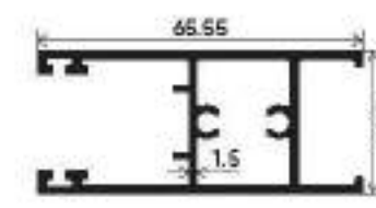
Top & Bottom DGU Shutter Section Number : V-3116 Weight (kg/mt) : 1.079
