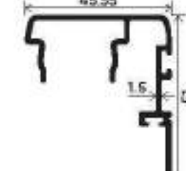
INTERLOCK
