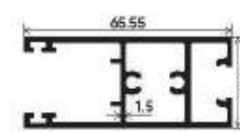
Top & Bottom S. G. Shutter Section Number : V-3112 Weight (kg/mt) : 1.079
