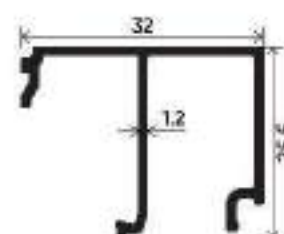
CLIP
