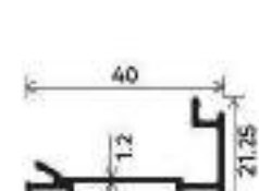
ECO CLIP
