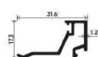
INTERLOCK CLIP
