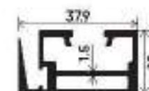
Slim Interlock S. G. Section Number : V-3121 Weight (kg/mt) : 0.683
