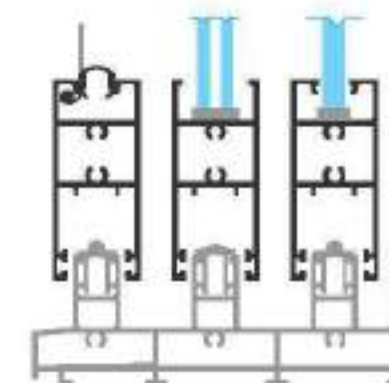
Slim Interlock SG & DGU
