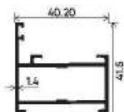
ECO FRAME
