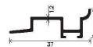
INTERLOCK CLIP
