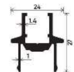
CLIP
