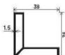
38 X 38 Angle Section Number : V-2740 Weight (kg/12') : 2.038
