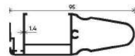
INTERLOCK
