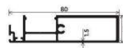
INTERLOCK
